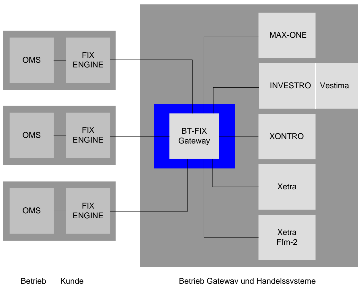
Abbildung 1-1: Systemüberblick
