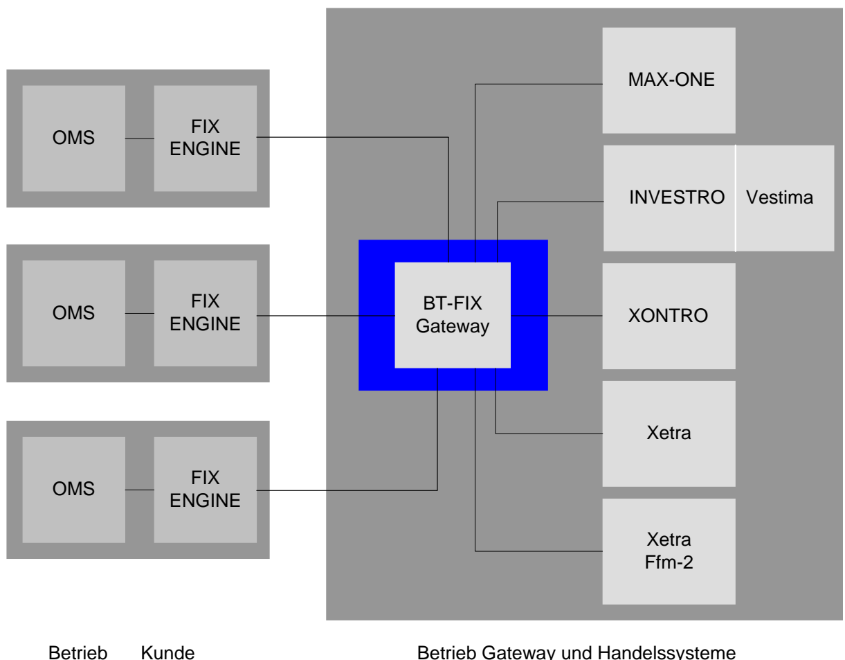
Abbildung 1-1: Systemüberblick
